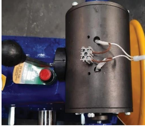
Şekil 7.2. 198 v DC Fren Bağlantısı
