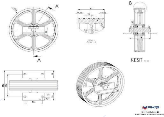
Şekil 19.4. Saptırma Kasnağının Gösterimi
